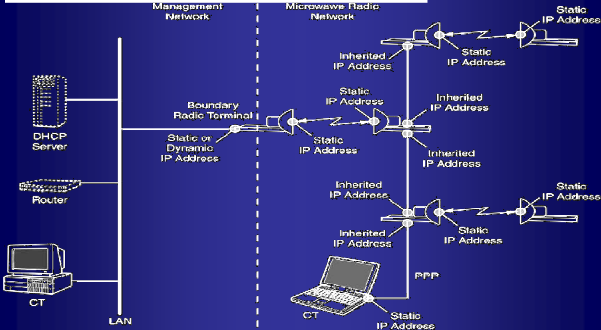
Beispiel eines Richtfunk-Netzwerkes mit statischen (festen) IP-Adressen
